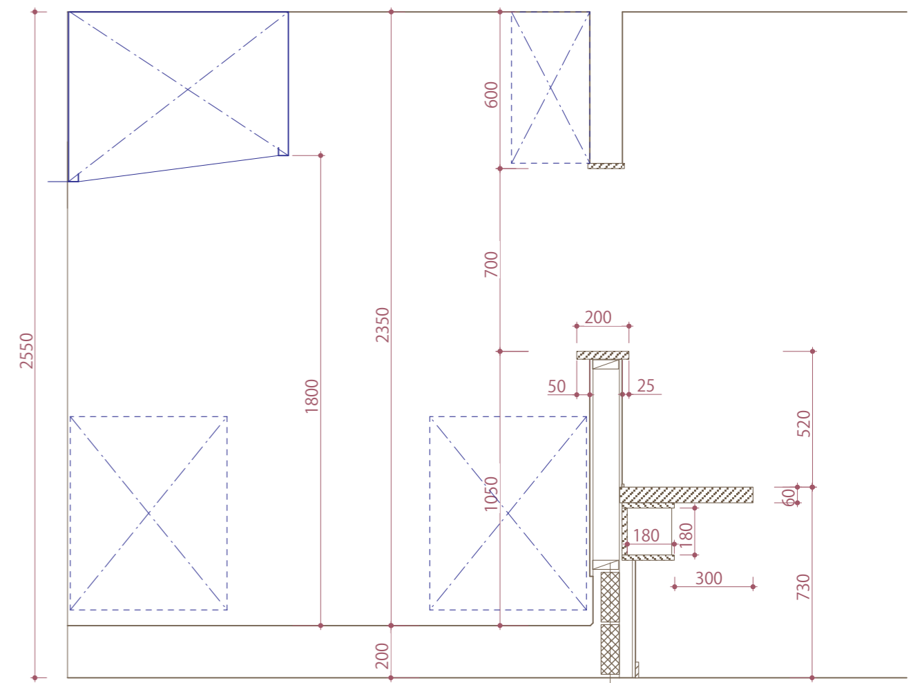
断面図 S 1:20
